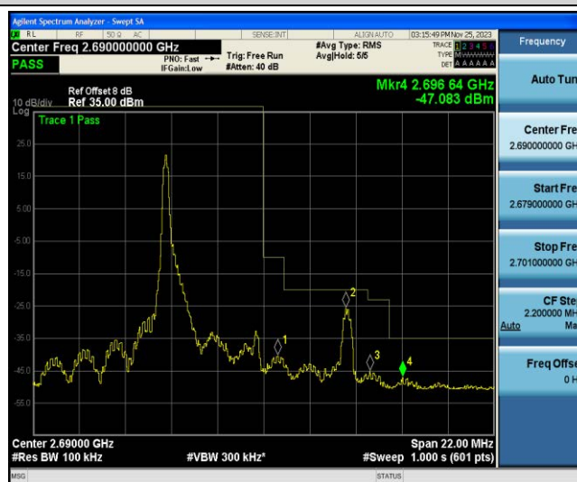
Band41-5MHz-16QAM-41565-1RB#24
