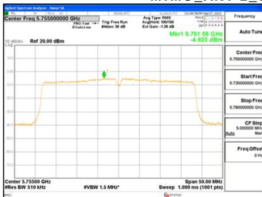
MIMO_ANT 1_802.11ac_VHT40_UNII-3
