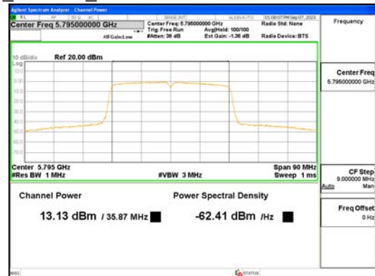
MIMO_ANT 1_802.11ac_VHT40_UNII-3
