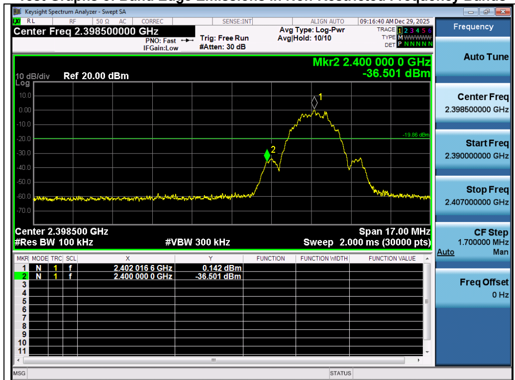
Test_Graph_SRD_ANT1_2402_Lower Band Edge Emissions
