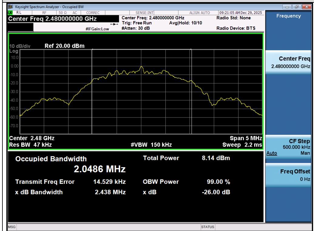
Test_Graph_SRD_ANT1_2480_OBW
