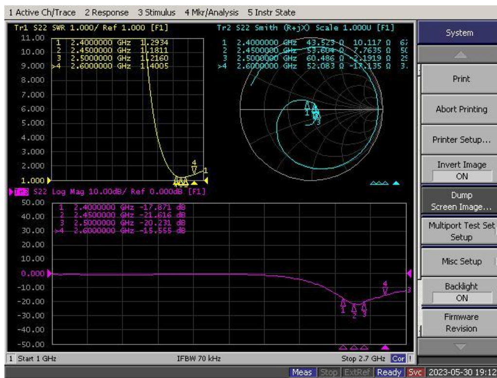
图 1 Smith Chart
