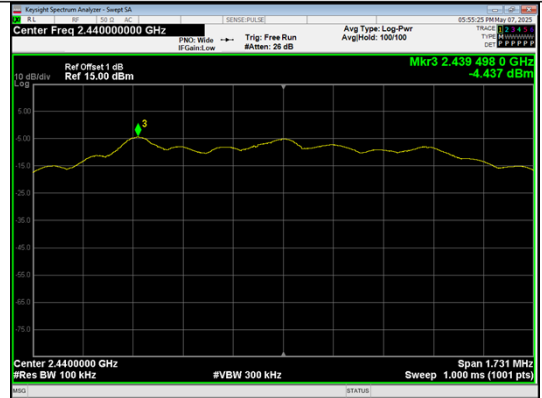
In-Band Reference Level BLE 2M_Channel 19 1 1 2 2 3 3 4 4 5 5 6 6 7 7 8 8 9 9 10 10 11 11 12 12 13 13 14 14 15 15 16 16 17 17 18 18 19 19 20 20 21 21 22 22 23 23 24 24 25 25 26 26 27 27 28 28 29 29 30 30 31 31 32 32 33 33 34 34 35 35 36 36 37 37 38 38 39 39 40 40 41 41 42 42 43 43 44 44 45 45 46 46 47 47 48 48 49 49 50 50 51 51 52 52 53 53 54 54 55 55 56 56 57 57 58 58 59 59 60 60 61 61 62 62 63 63 64 64 65 65 66 66 67 67 68 68 69 69 70 70 71 71 72 72 73 73 74 74 75 75 76 76 77 77 78 78 79 79 80 80 81 81 82 82 83 83 84 84 85 85 86 86 87 87 88 88 89 89 90 90 91 91 92 92 93 93 94 94 95 95 96 96 97 97 98 98 99 99 100 100
