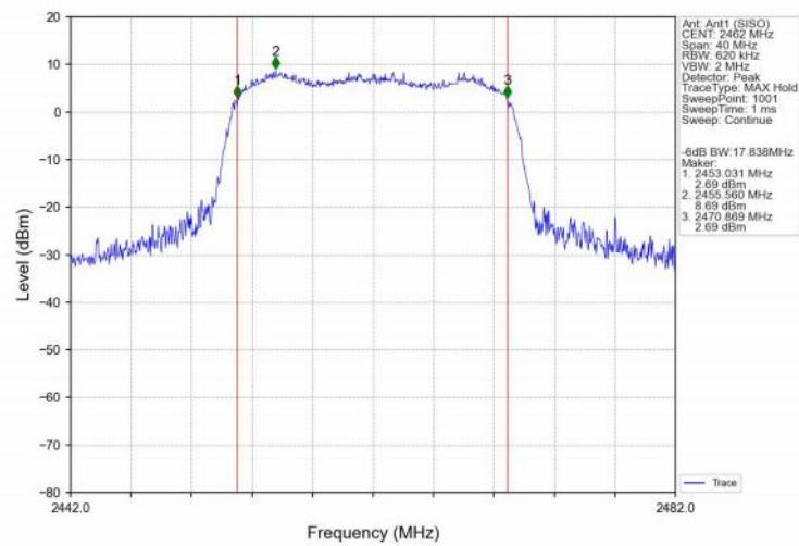
802.11n(HT20) HCH 2462MHz Ant1 (SISO) NTN
