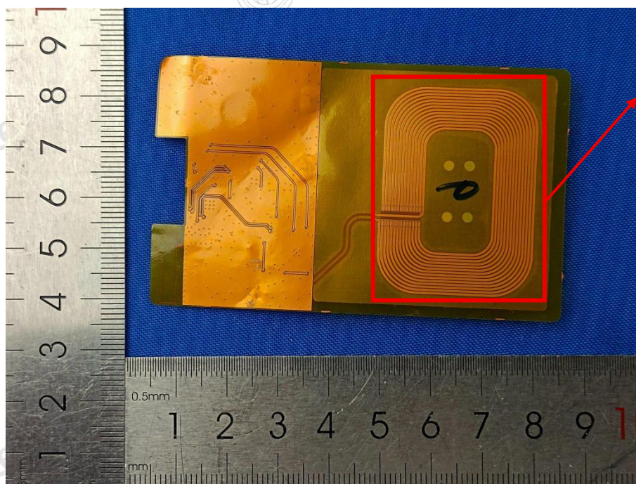
WPT RX
