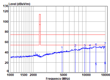
2.4G_SRD_TX_LOW_Horizontal
