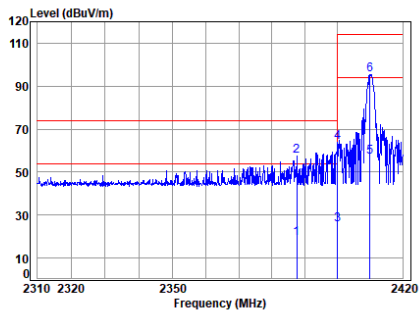
2.4G_SRD_LOW_TX_Horizontal
