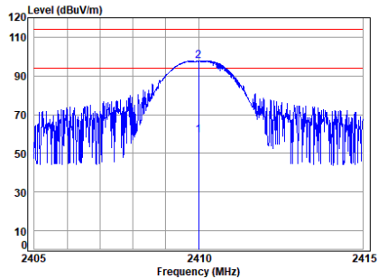
2.4G_SRD_LOW_TX_Horizontal
