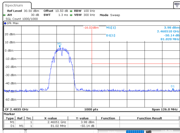
802.11b_2462MHz
