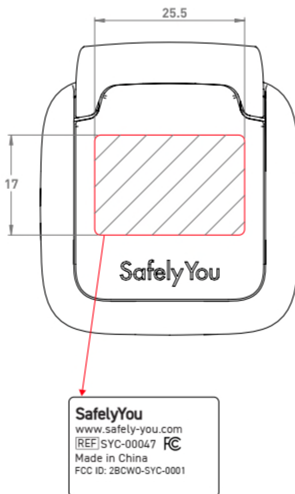
Figure 2 – Halo™ Pendant
