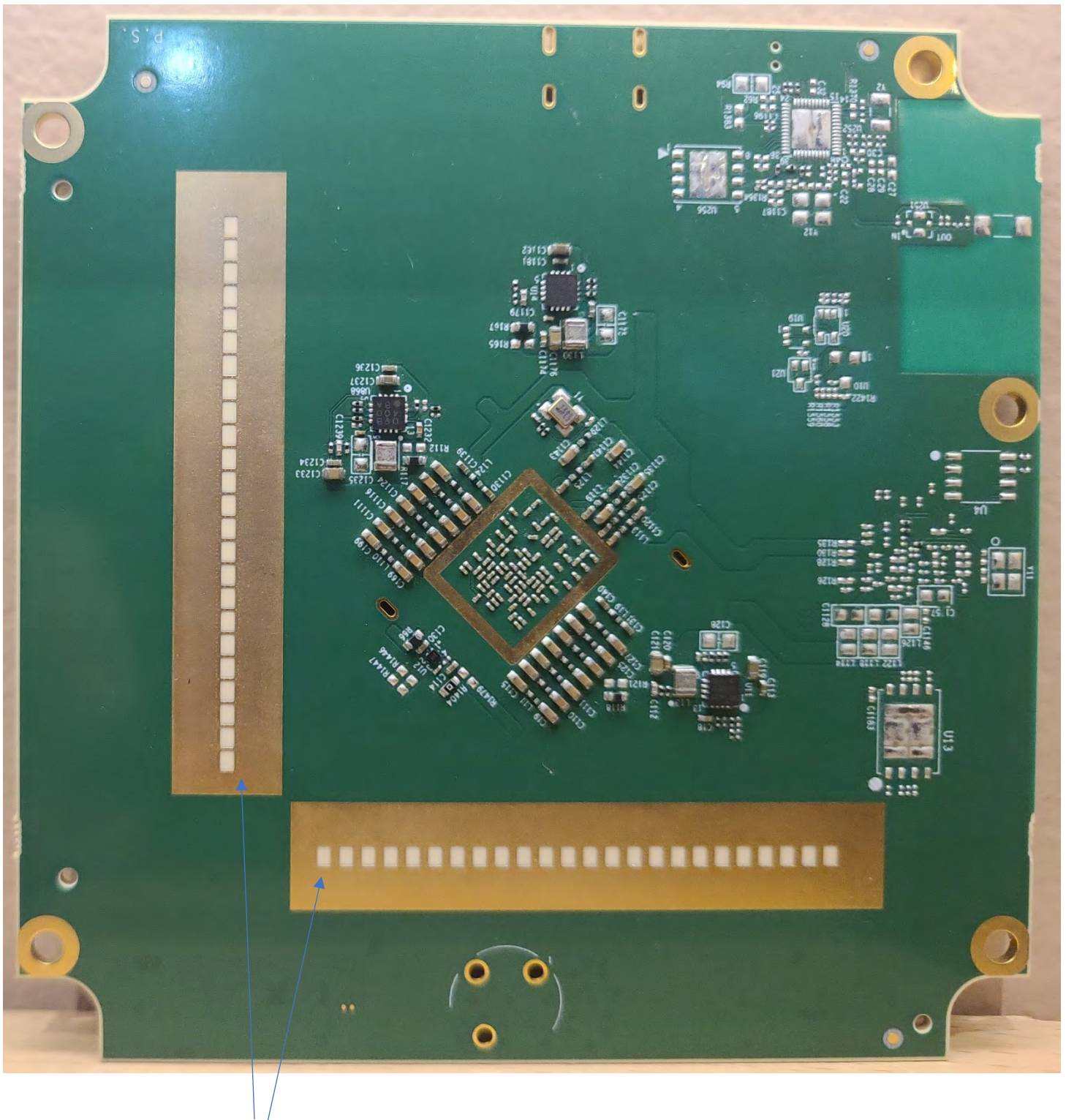
ANTENNA ARRAY
