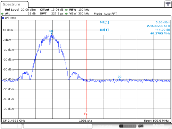
IEEE 802.11b Right Side
