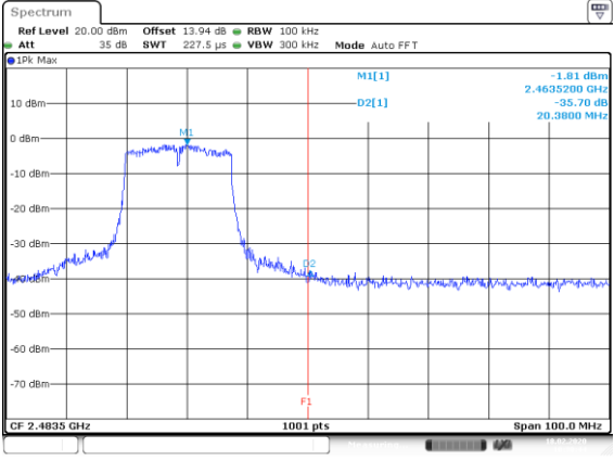
IEEE 802.11n HT20 Right Side
