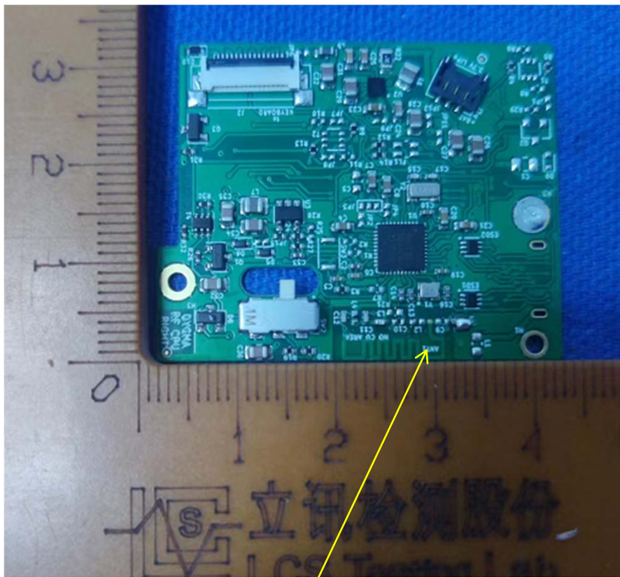
Antenna
