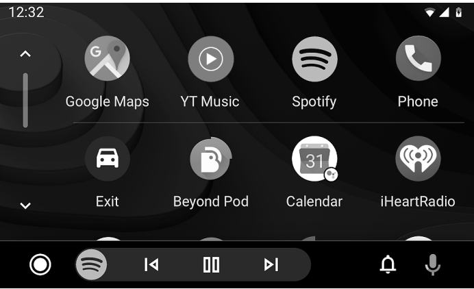
Android Auto
