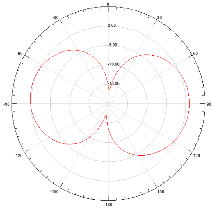
H-Plan
