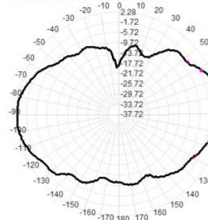
2450.0MHz Total(E2-YZ), Max= 2.28dBi
