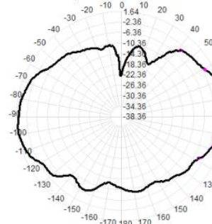
2500.0MHz Total(E2-YZ), Max= 1.64dBi
