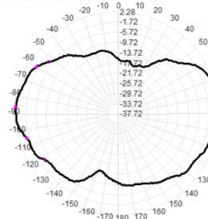
2450.0MHz Total(E1-XZ), Max= 2.21dBi
