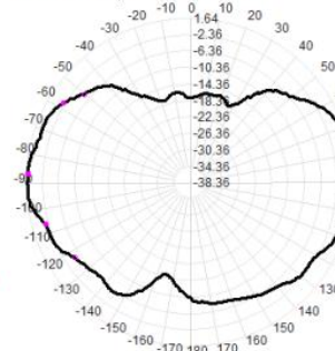
2500.0MHz Total(E1-XZ), Max= 1.25dBi
