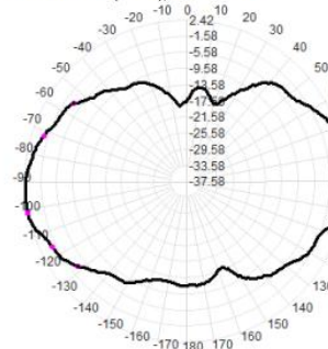
2400.0MHz Total(E2-YZ), Max= 2.37dBi
