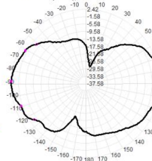
2400.0MHz Total(E1-XZ), Max= 2.30dBi
