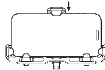
4. 调节左、右侧固定扣滑块贴合手机，往下压紧顶部固定扣滑块夹紧手机。
