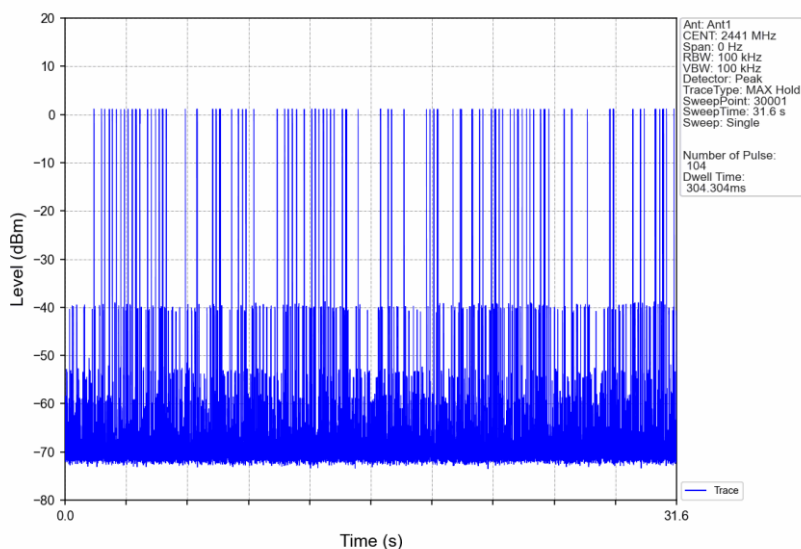
Pi/4DQPSK_2DH5_HOPP_Ant1_NTNV
