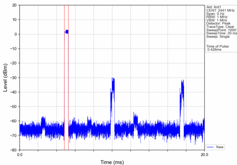
Pi/4DQPSK_2DH1_HOPP_Ant1_NTNV
