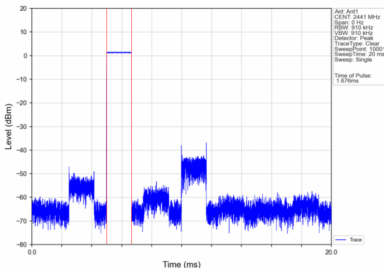
GFSK_DH3_HOPP_Ant1_NTNV
