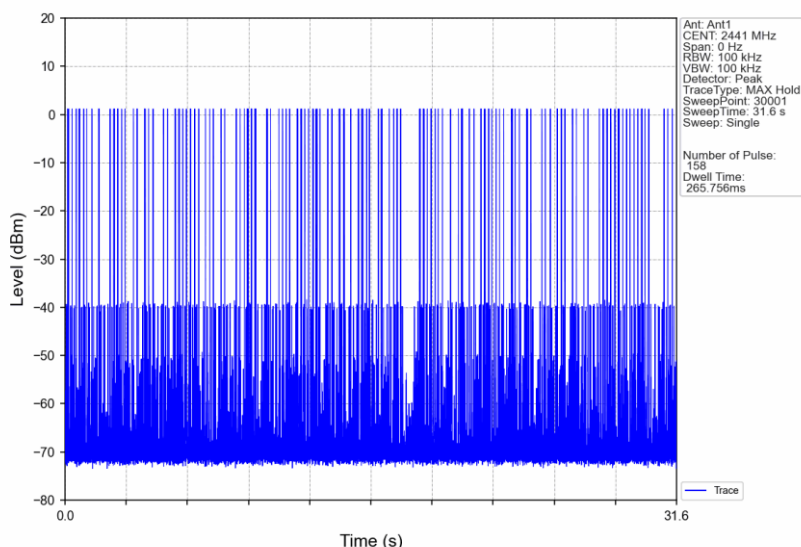
Pi/4DQPSK_2DH3_HOPP_Ant1_NTNV
