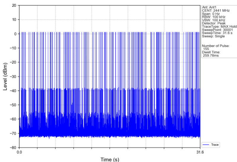
GFSK_DH3_HOPP_Ant1_NTNV
