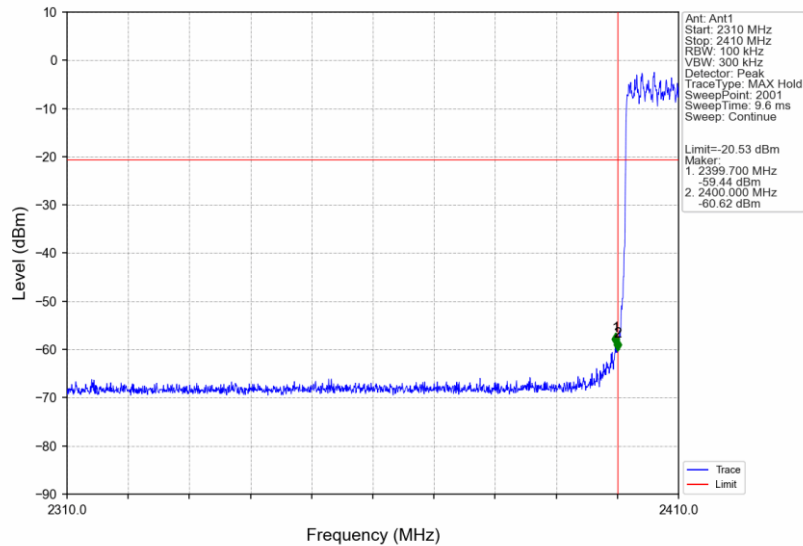
Pi/4DQPSK_2DH5_HOPP_Ant1_NTNV
