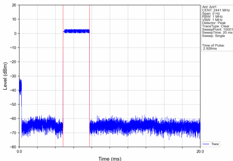
Pi/4DQPSK_2DH5_HOPP_Ant1_NTNV
