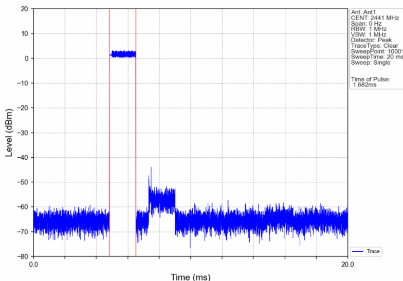
Pi/4DQPSK_2DH3_HOPP_Ant1_NTNV
