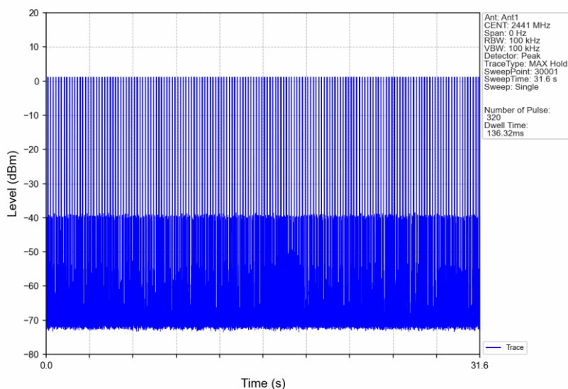
Pi/4DQPSK_2DH1_HOPP_Ant1_NTNV
