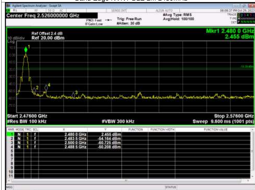
Band Edge NVNT BLE 2M 2480MHz
