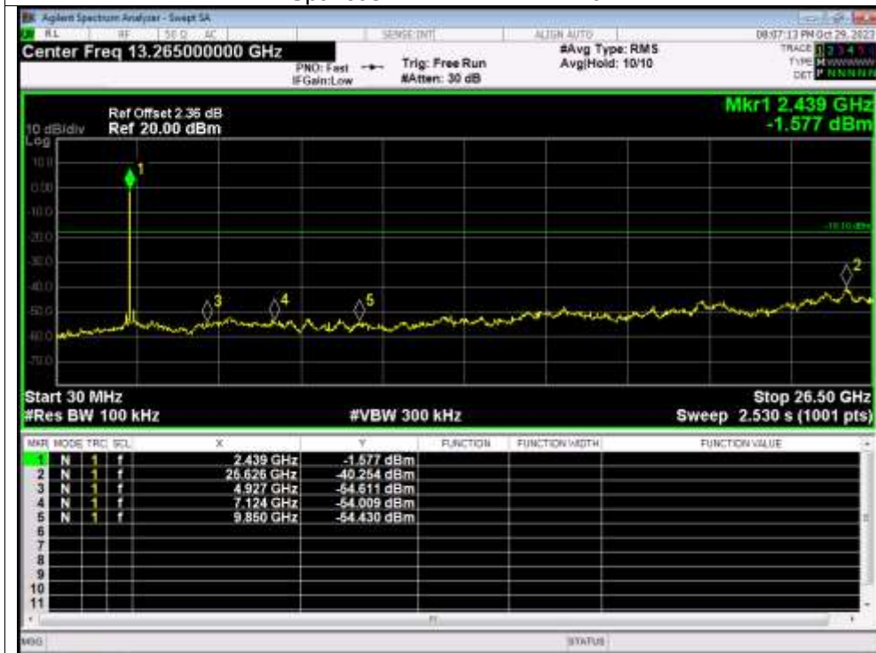
Tx. Spurious NVNT BLE 2M 2440MHz
