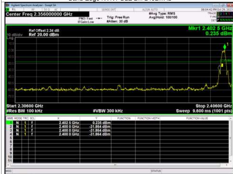
Band Edge NVNT BLE 2M 2402MHz
