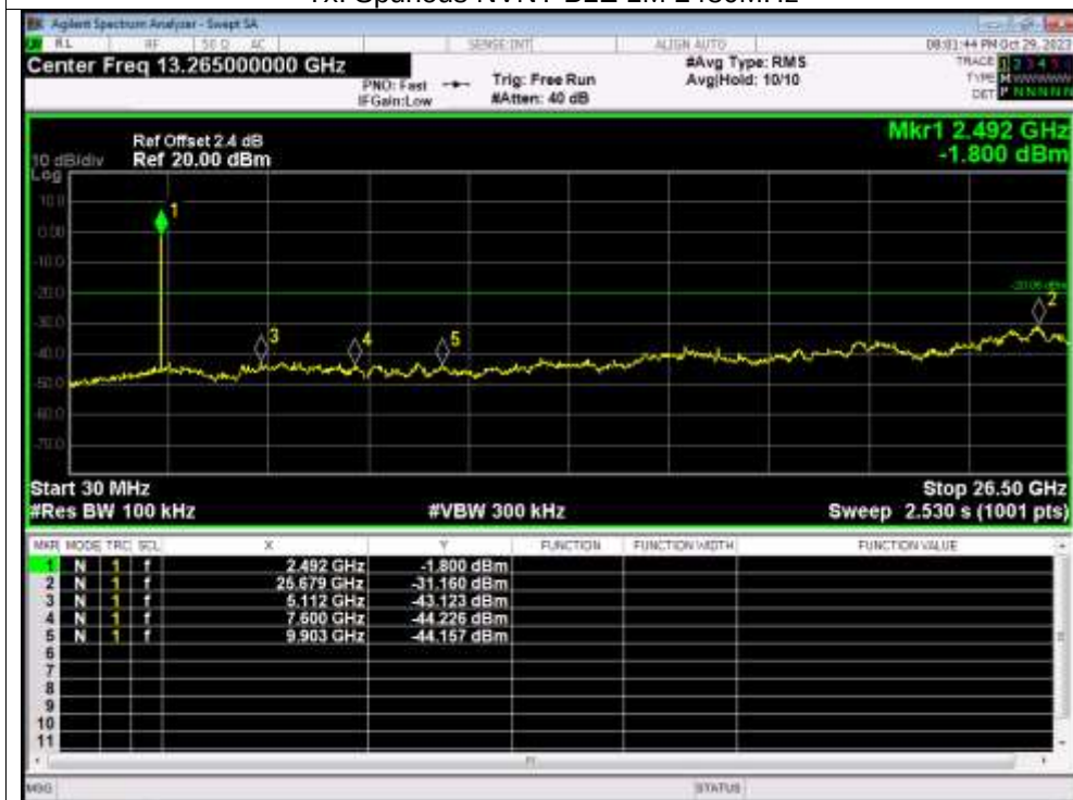
Tx. Spurious NVNT BLE 1M 2480MHz
