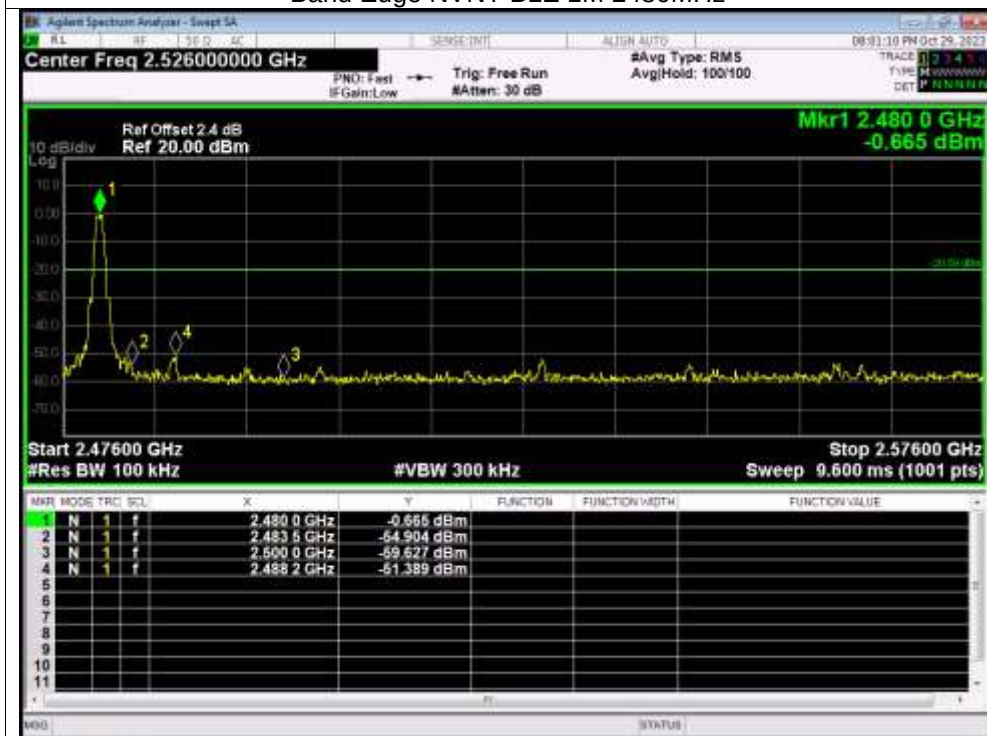
Band Edge NVNT BLE 1M 2480MHz
