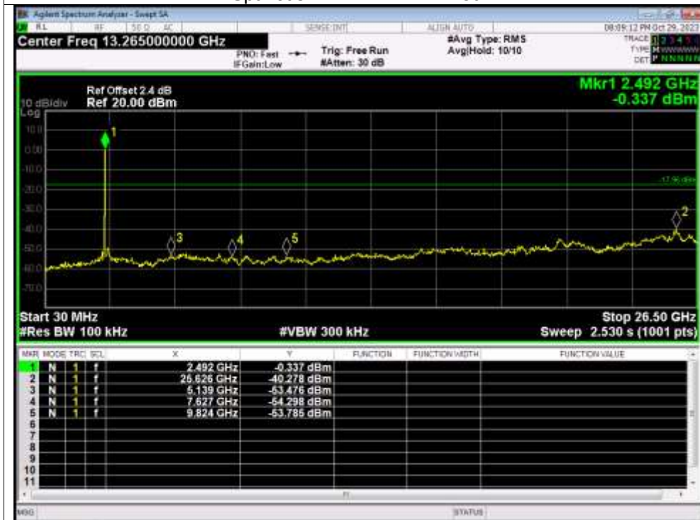
Tx. Spurious NVNT BLE 2M 2480MHz
