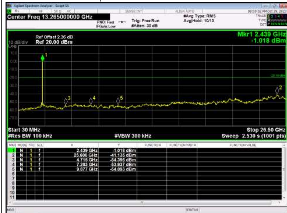
Tx. Spurious NVNT BLE 1M 2440MHz
