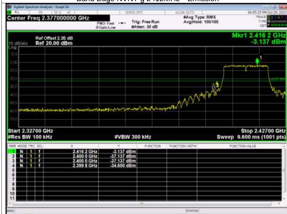
Band Edge NVNT g 2412MHz Emission
