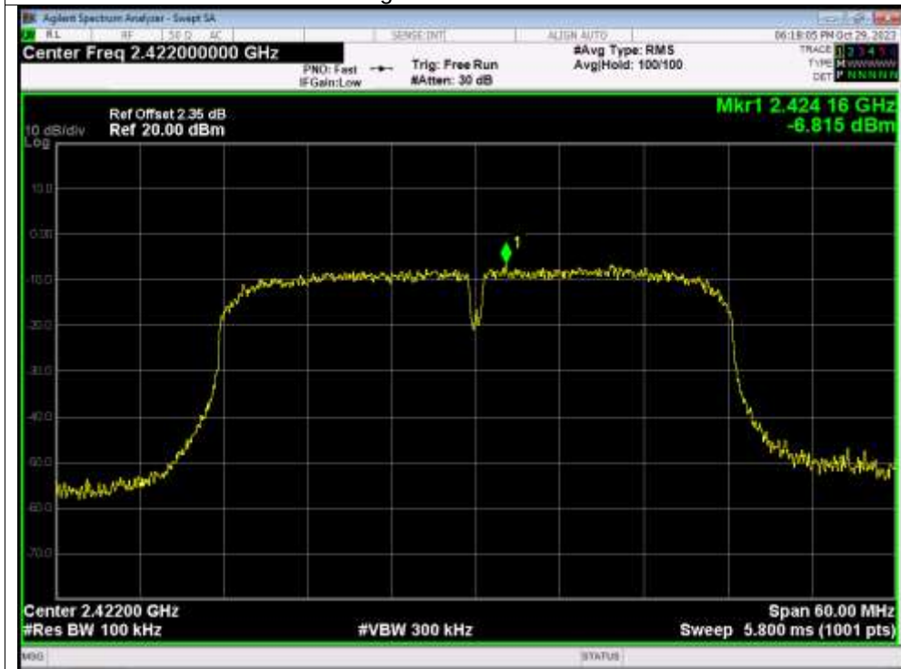
Band Edge NVNT n40 2422MHz Emission
