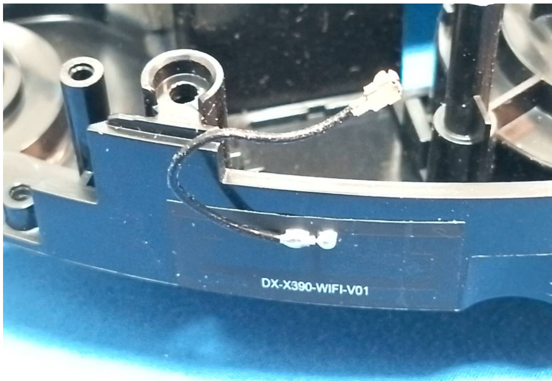
Bluetooth&Wifi Antenna
