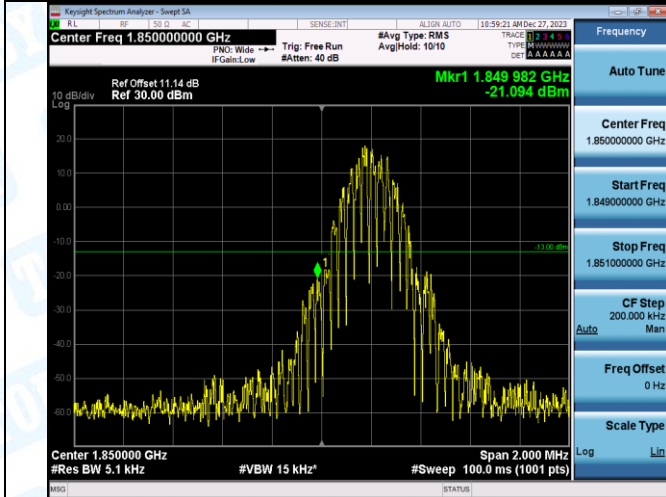
GPRS1900-512-0-PASS
