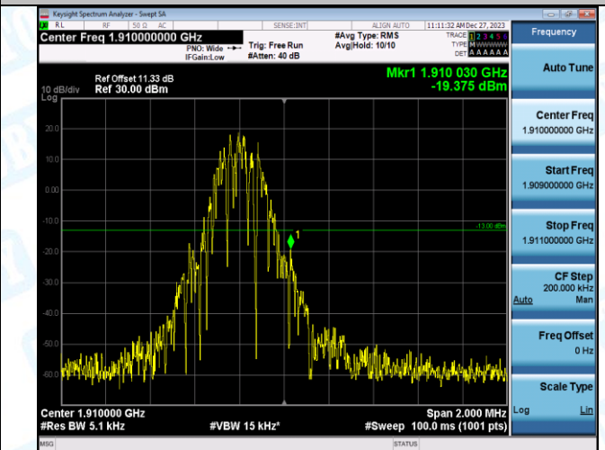
EGPRS1900-810-2-PASS
