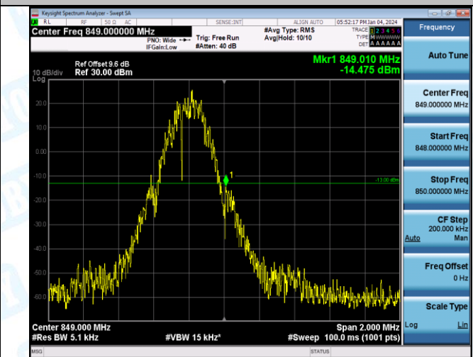
GSM850-251-5-PASS
