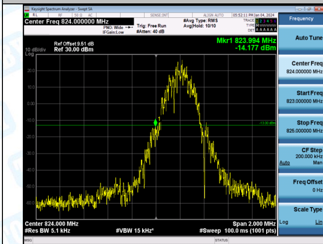
GSM850-128-5-PASS
