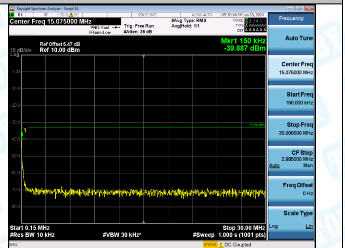
Band4-1413-4-1000~20000MHz-PASS
