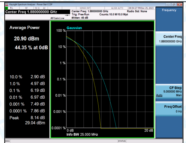
Band2-20MHz-16QAM-19100-1RB#0-PASS
