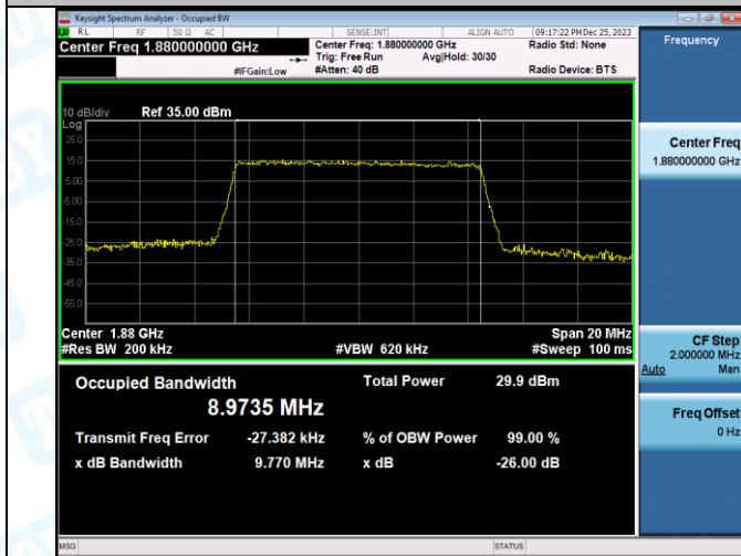
Band2-10MHz-16QAM-18900-50RB#0-PASS
