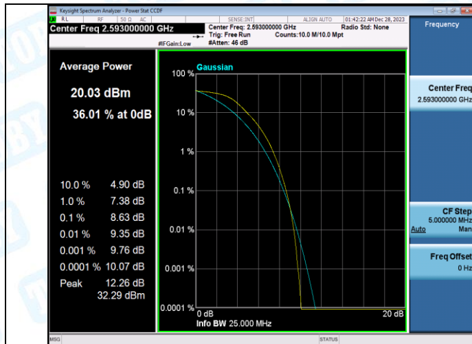
Band41-20MHz-QPSK-41490-1RB#0-PASS
