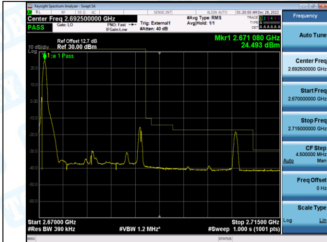
Band41_20MHz_QPSK_41490_1RB#99
