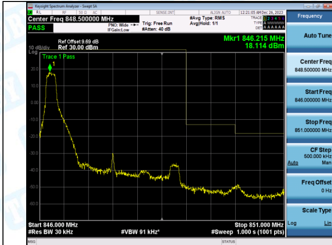
Band5_3MHz_QPSK_20635_1RB#14
