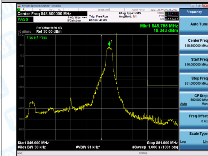
Band5_3MHz_QPSK_20635_15RB#0
