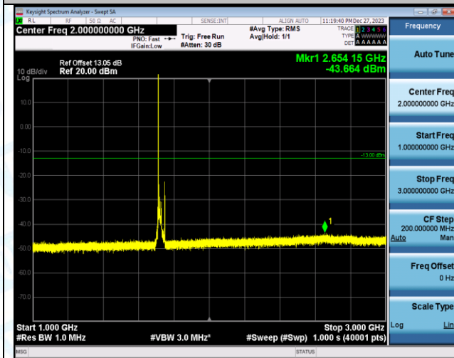
Band66_20MHz_QPSK_132072_1RB#0_2.000000000 GHz
