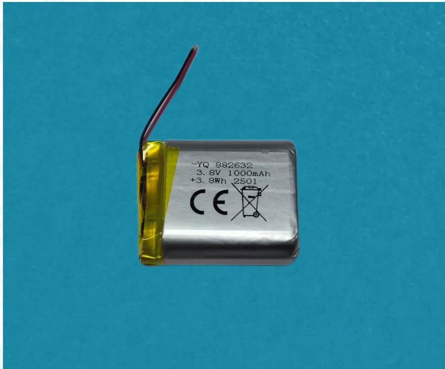
Photo 13 Battery parameters
