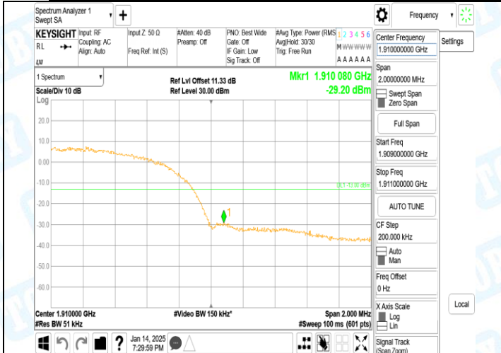
Band2-9538-3-PASS
