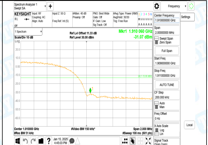
Band2-9538-3-PASS
