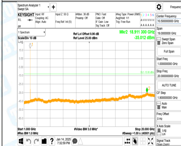
Band2-9538-1-1000~20000MHz-PASS
