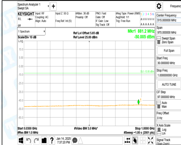
Band2-9538-3-30~1000MHz-PASS
