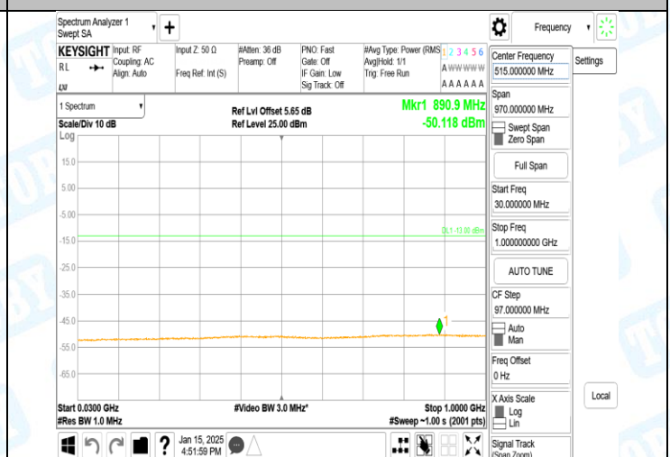
Band2-9538-2-30~1000MHz-PASS
