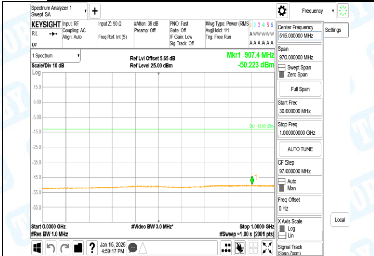
Band2-9538-5-30~1000MHz-PASS
