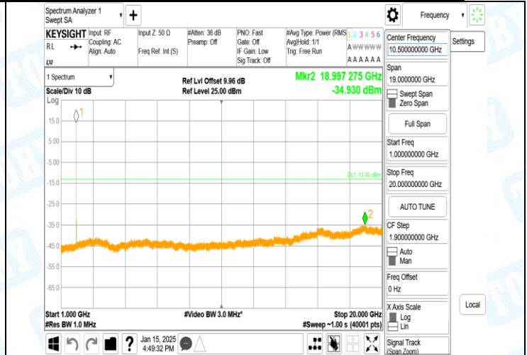
Band2-9538-1-1000~20000MHz-PASS
