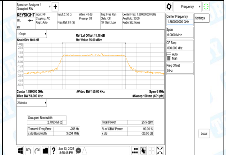
Band2-3MHz-QPSK-18900-15RB#0-PASS
