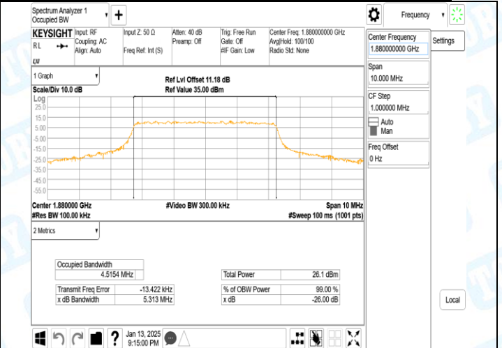
Band2-5MHz-QPSK-18900-25RB#0-PASS
