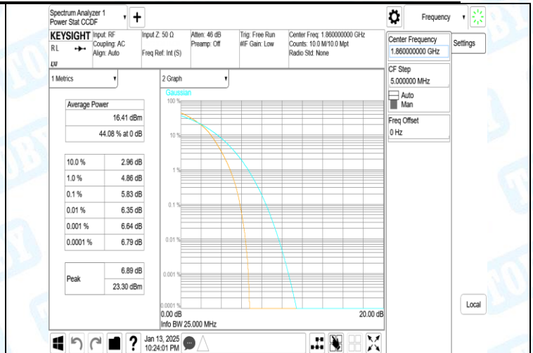
Band2-20MHz-16QAM-18700-100RB#0-PASS
