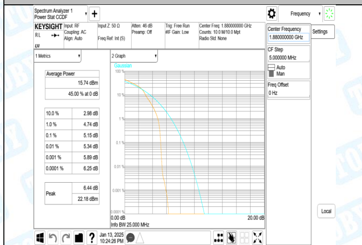
Band2-20MHz-16QAM-18900-1RB#0-PASS
