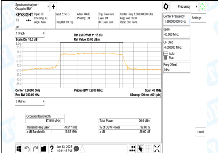
Band2-20MHz-QPSK-18700-100RB#0-PASS
