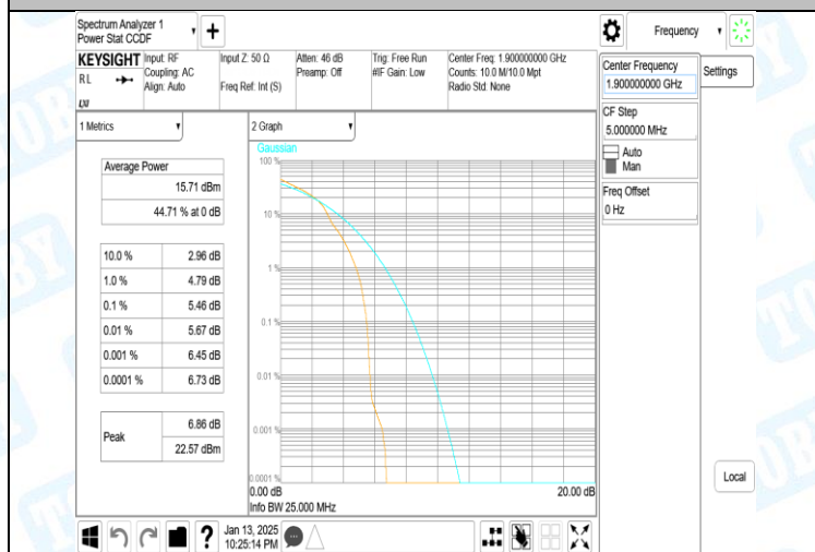
Band2-20MHz-16QAM-19100-1RB#0-PASS
