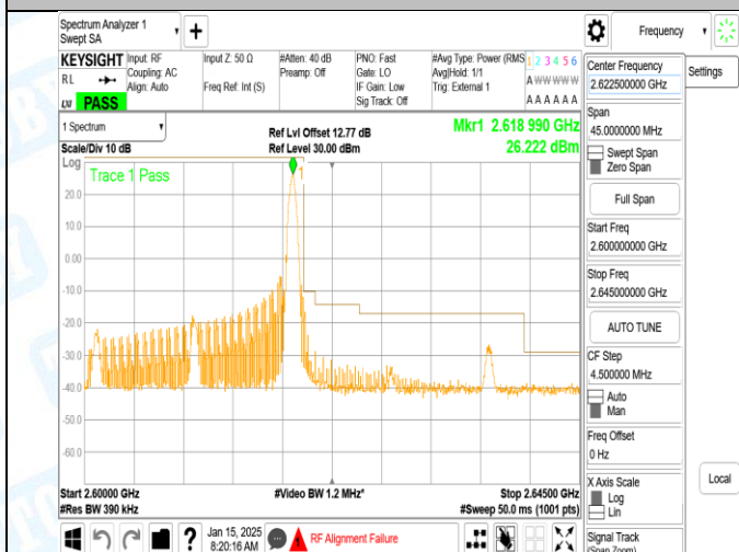
Band38_20MHz_QPSK_38150_1RB#99
