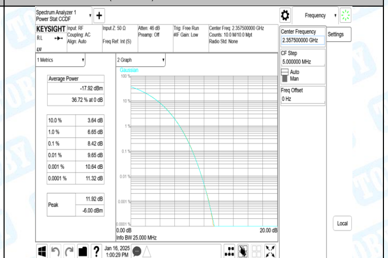
40(2350-2360)-5MHz-QPSK-39225-25RB#0-PASS
