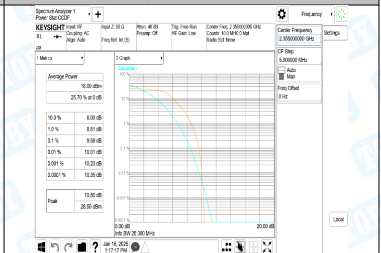
40(2350-2360)-10MHz-QPSK-39200-50RB#0-PASS
