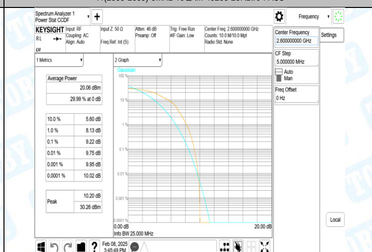
41(2555-2655)-5MHz-16QAM-40690-25RB#0-PASS
