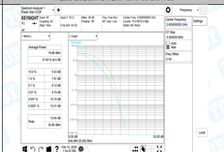
41(2555-2655)-20MHz-16QAM-40690-100RB#0-PASS
