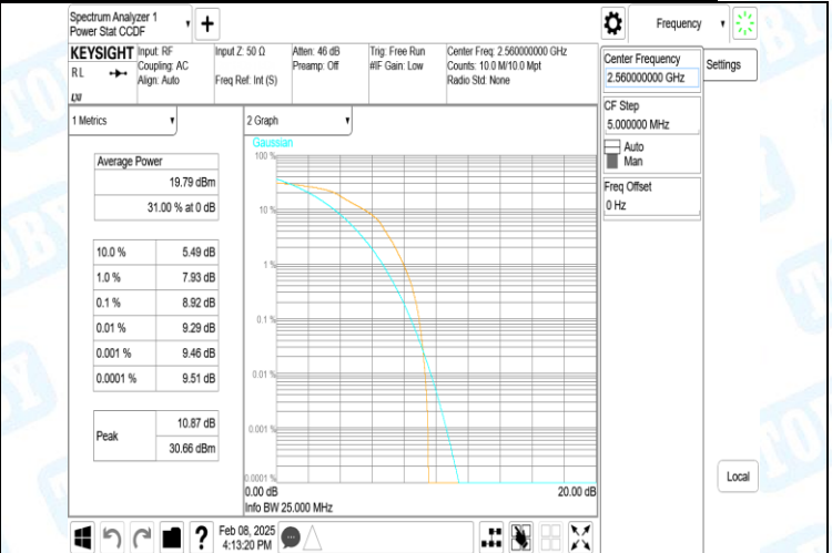
41(2555-2655)-10MHz-16QAM-40290-50RB#0-PASS
