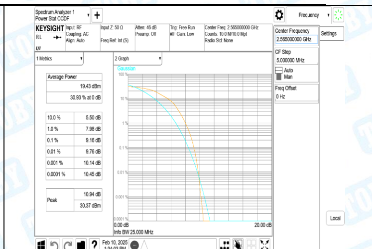
41(2555-2655)-20MHz-16QAM-40340-100RB#0-PASS
