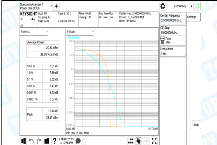
41(2555-2655)-10MHz-16QAM-40290-1RB#0-PASS
