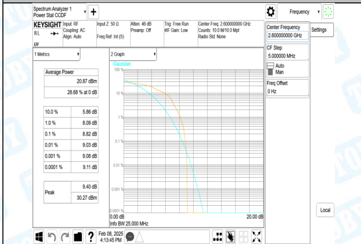
41(2555-2655)-10MHz-16QAM-40690-1RB#0-PASS
