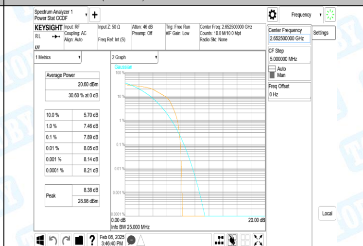
41(2555-2655)-5MHz-16QAM-41215-25RB#0-PASS
