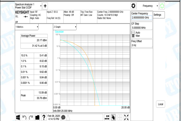
41(2555-2655)-10MHz-16QAM-40690-50RB#0-PASS
