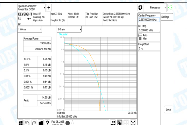
41(2555-2655)-5MHz-16QAM-40265-25RB#0-PASS
