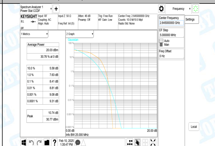
41(2555-2655)-20MHz-16QAM-41140-100RB#0-PASS
