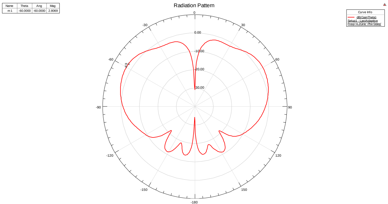
2D方向图
