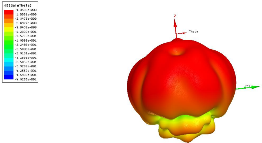
3D方向图
