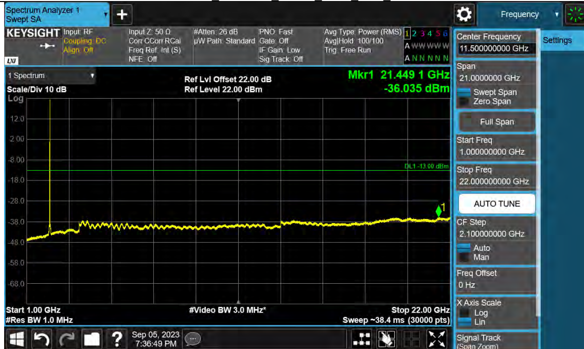
Band66_2179.8MHz_GMSK_SISO_Ant1_NTNV
