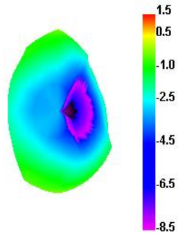
2450.000MHz
