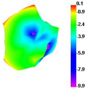
2500.000MHz E1
