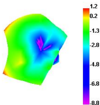
2400.000MHz E1
