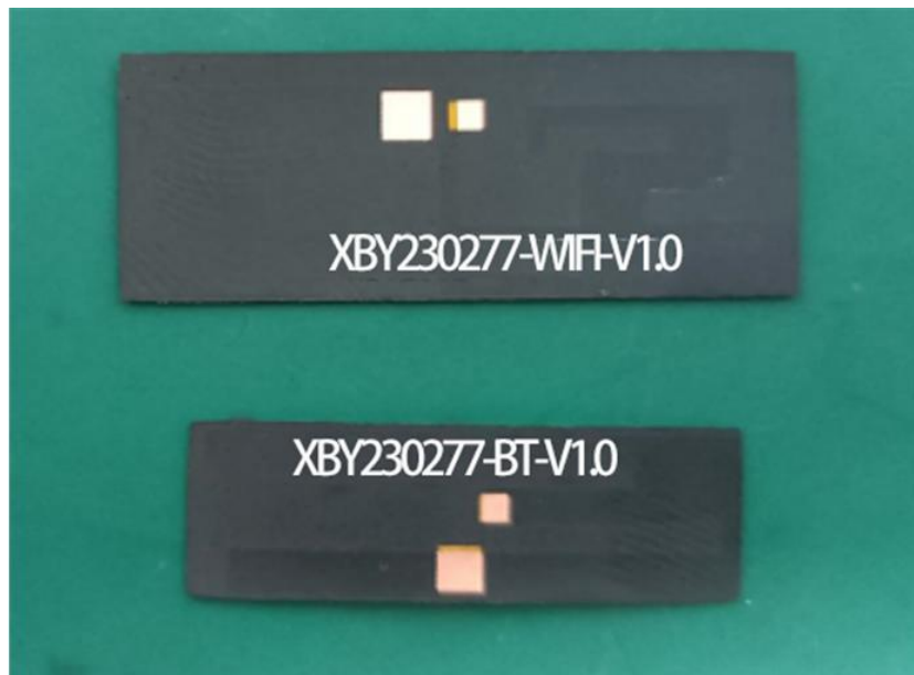
天线照片
