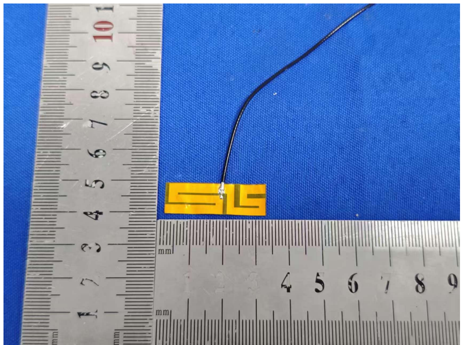
EUT Photo 8
