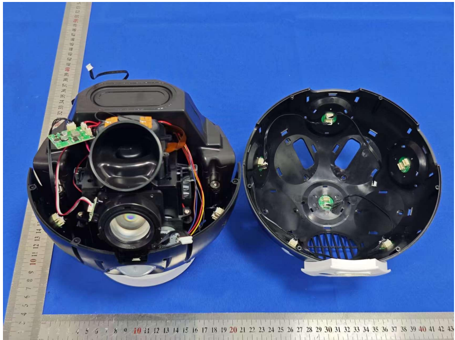
EUT Photo 1
