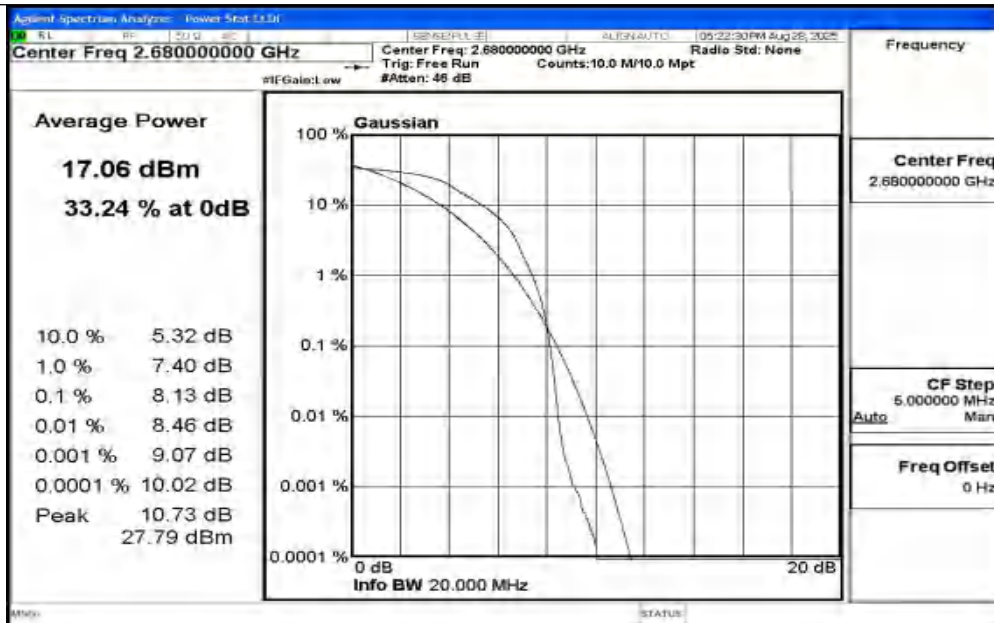
Band41-20MHz-QPSK-41490-1RB#0-PASS
