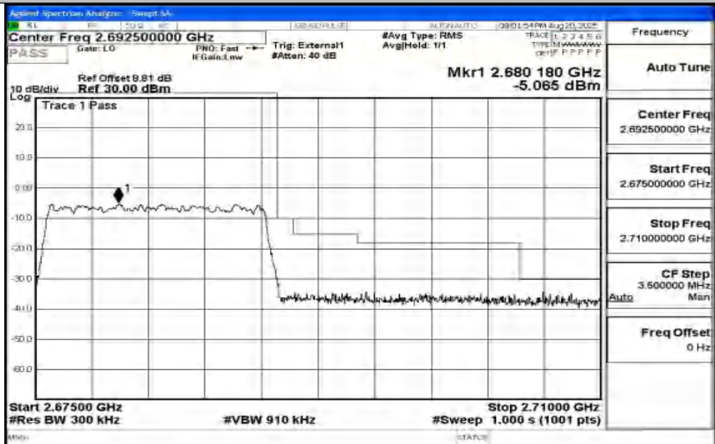
Band41_15MHz_QPSK_41515_75RB#0
