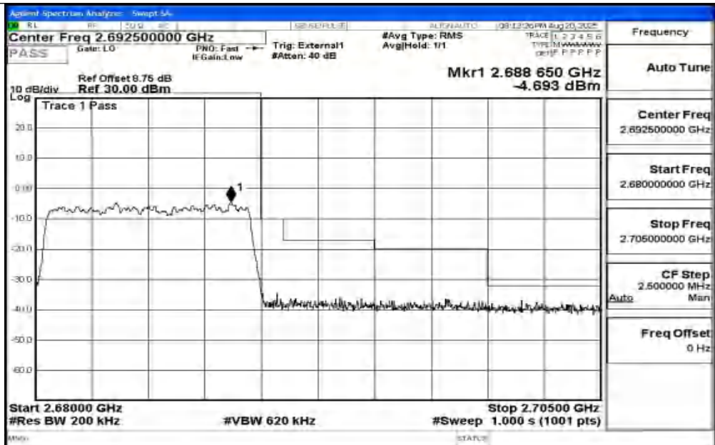
Band41_10MHz_QPSK_41540_50RB#0
