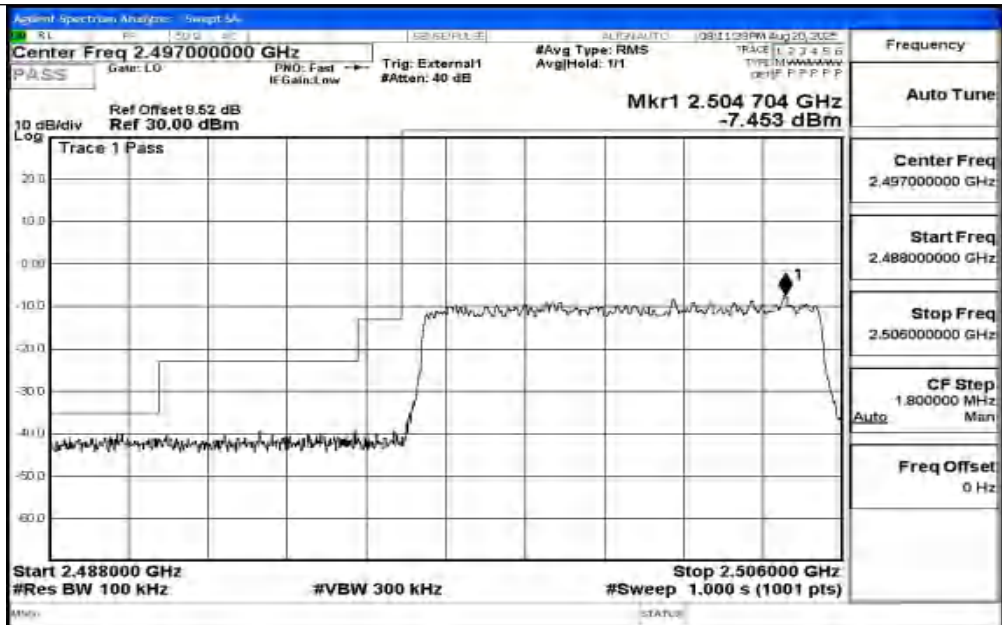
Band41_10MHz_QPSK_39700_50RB#0
