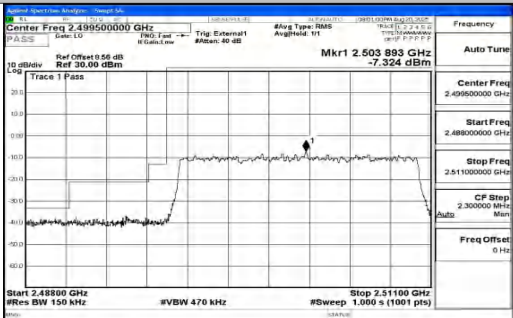
Band41_15MHz_QPSK_39725_75RB#0
