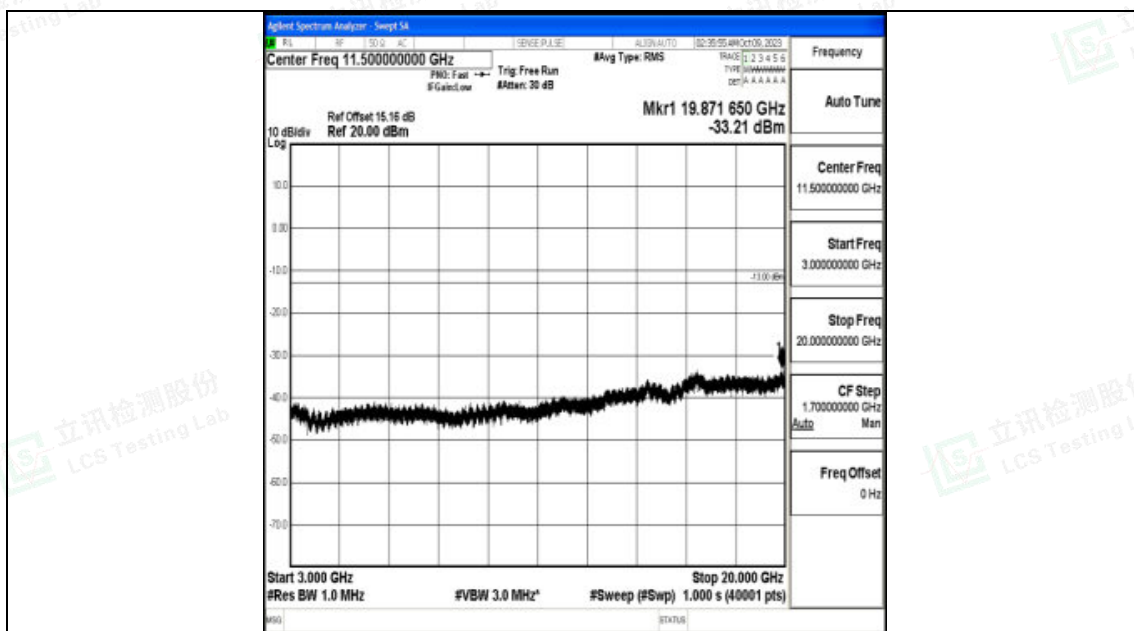
Band2 15MHz QPSK 19125 1RB#0 3000~20000 3000~20000
