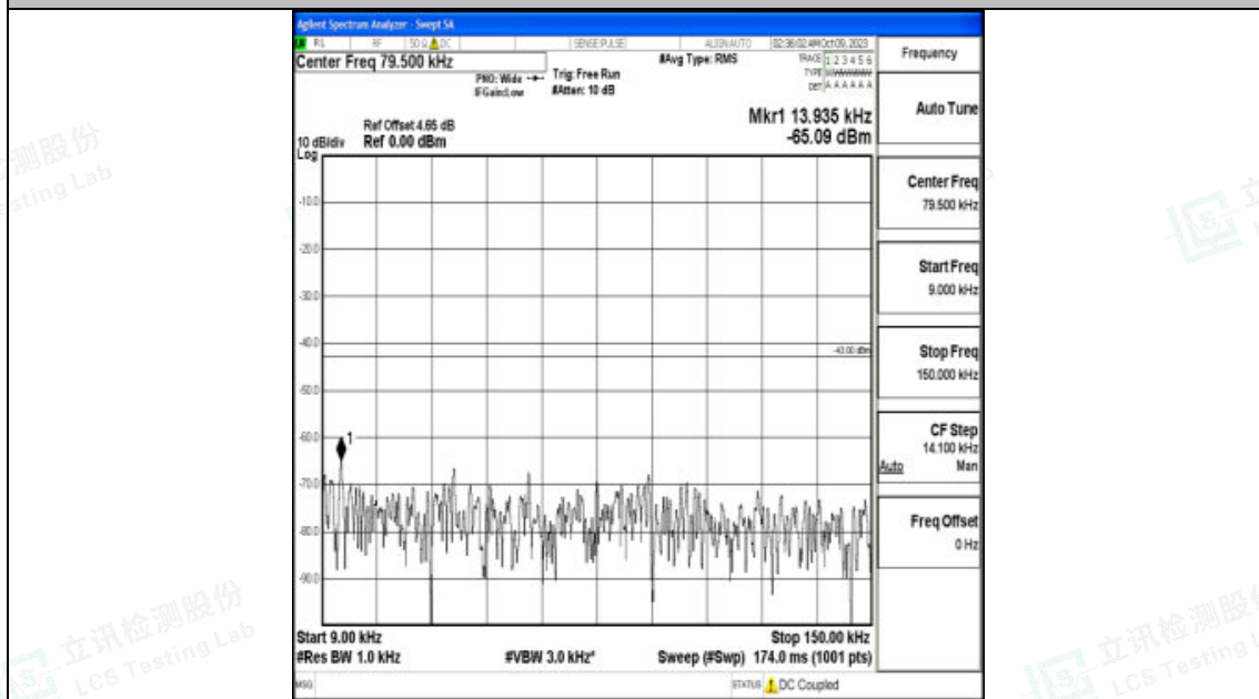
Band2 15MHz 16QAM 19125 1RB#0 0.009~0.15 0.009~0.15
