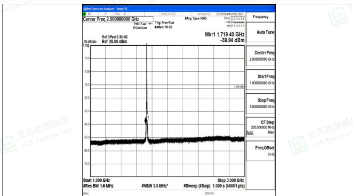
Band4 5MHz 16QAM 20175 1RB#0 1000~3000 1000~3000
