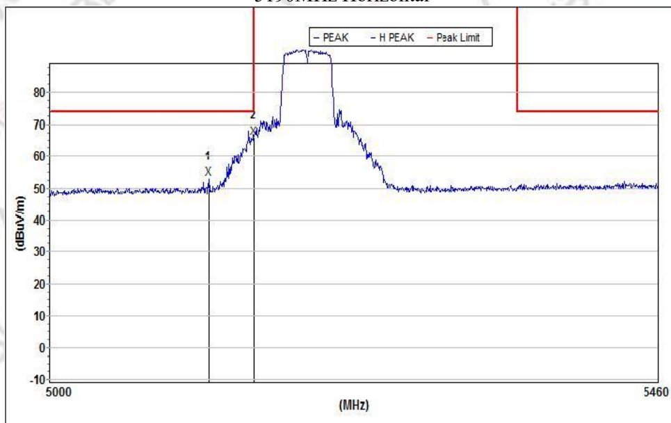
5190MHz Horizontal
