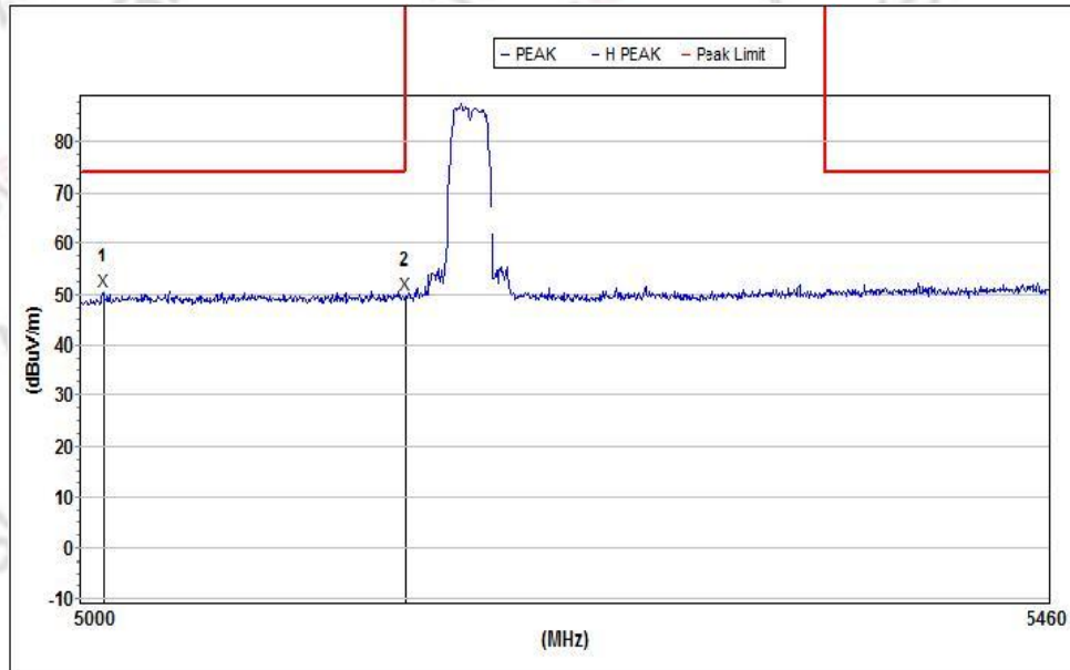
5180MHz Horizontal
