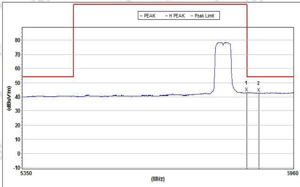
5795MHz Horizontal
