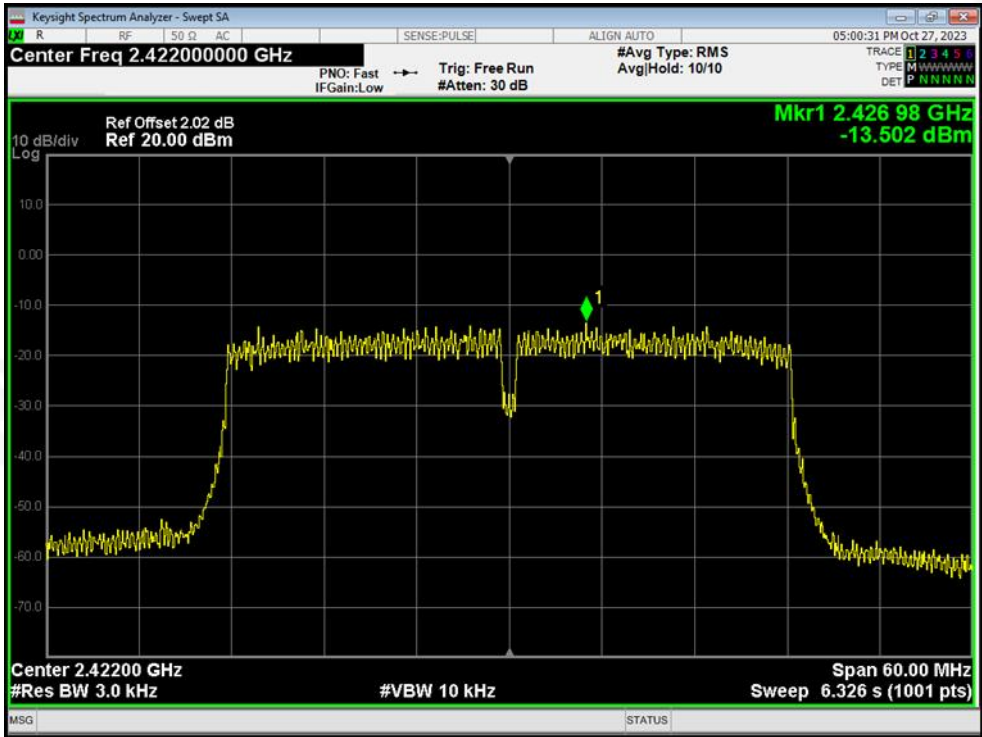
TX CH03
