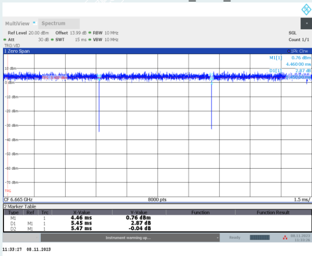
IEEE 802.11ax HE160_Ant1_6665MHz
