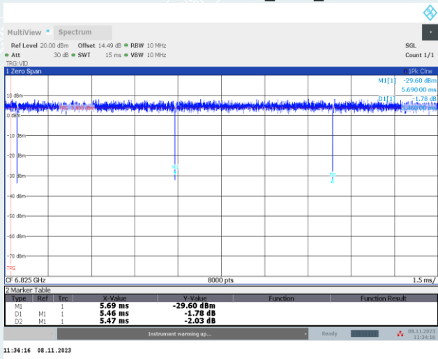
IEEE 802.11ax HE160_Ant1_6825MHz
