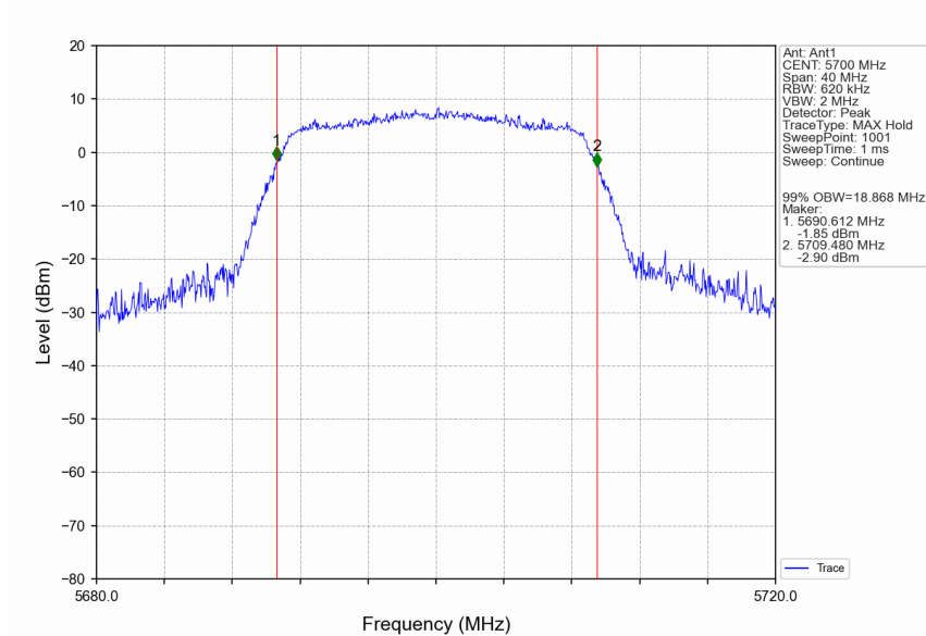
802.11ac(VHT20)_HCH_5700MHz_Ant1_NTNV
