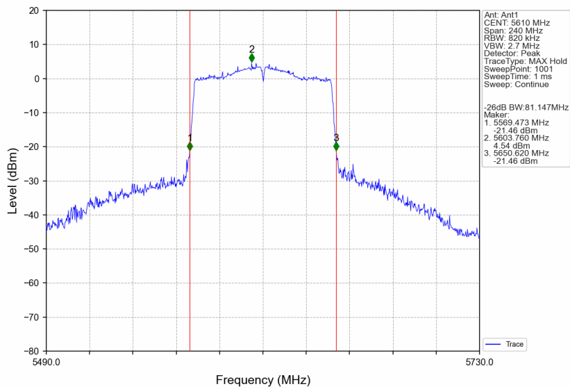
802.11ac(VHT80)_HCH_5610MHz_Ant1_NTNV
